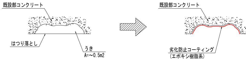
補修概要図
